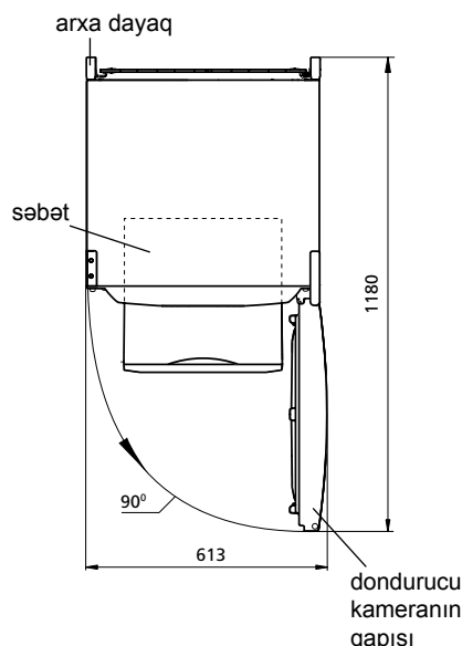
Şəkil 2 – Soyuducu (yuxarıdan görünüş)
