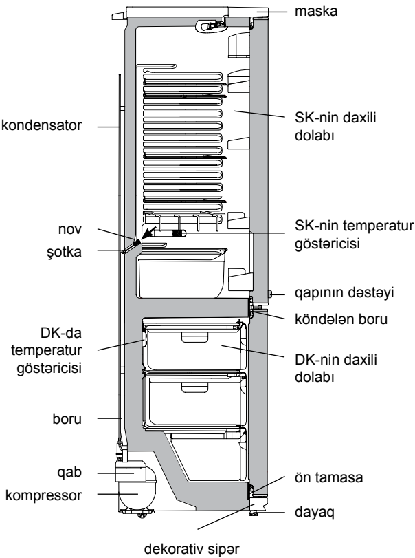
Şəkil 7 – SK-dən qar suyunun axma sistemi
