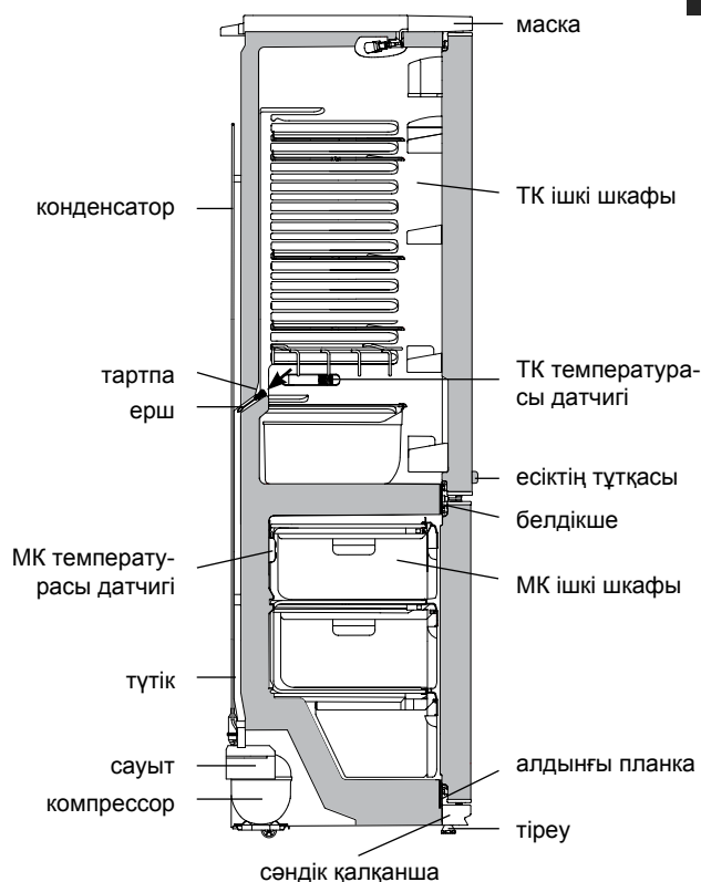
7 сурет – ТК еріген су ағызу схемасы
