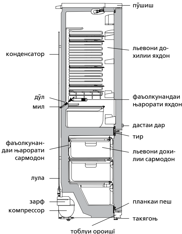
Расми 7 – Нақшаи партоби оби яхшудаи яхдон
