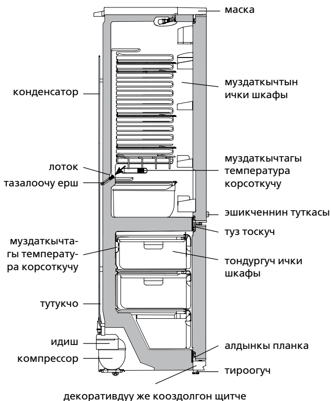
Сурот 7 – Муздаткычтан аккан суунун схемасы
