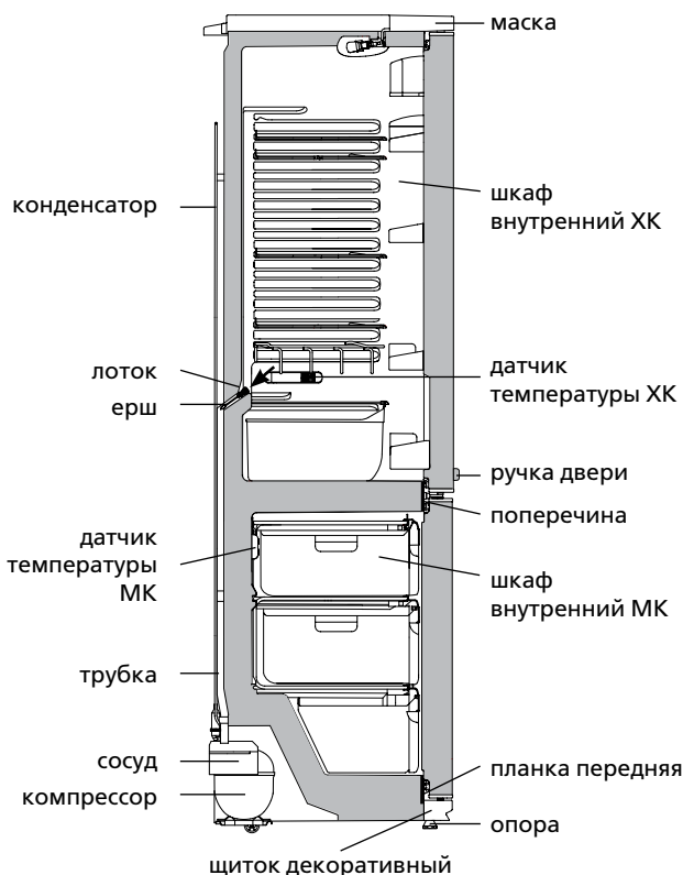
Рисунок 7 – Схема слива талой воды из ХК
